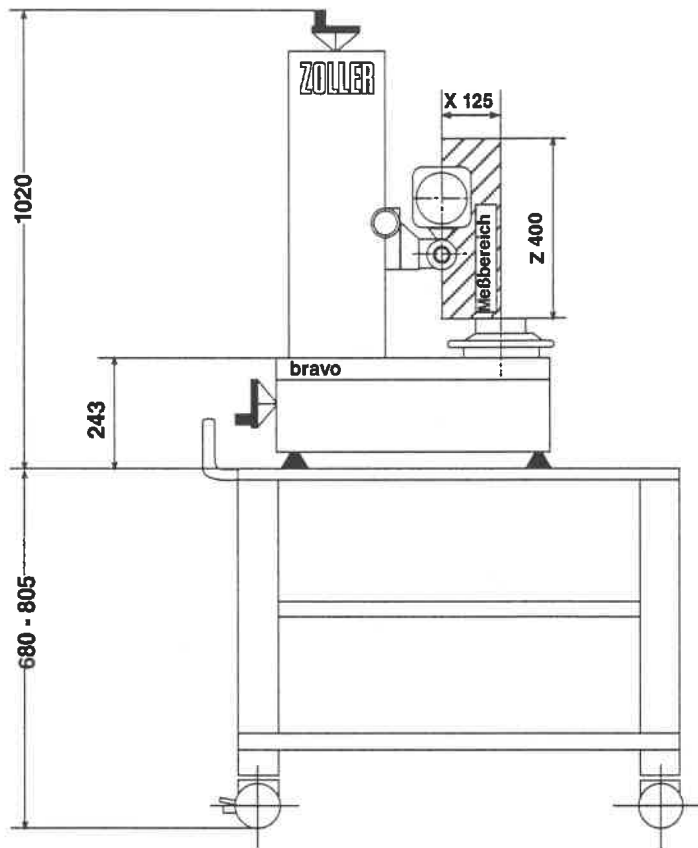
Gerätedraufsicht
