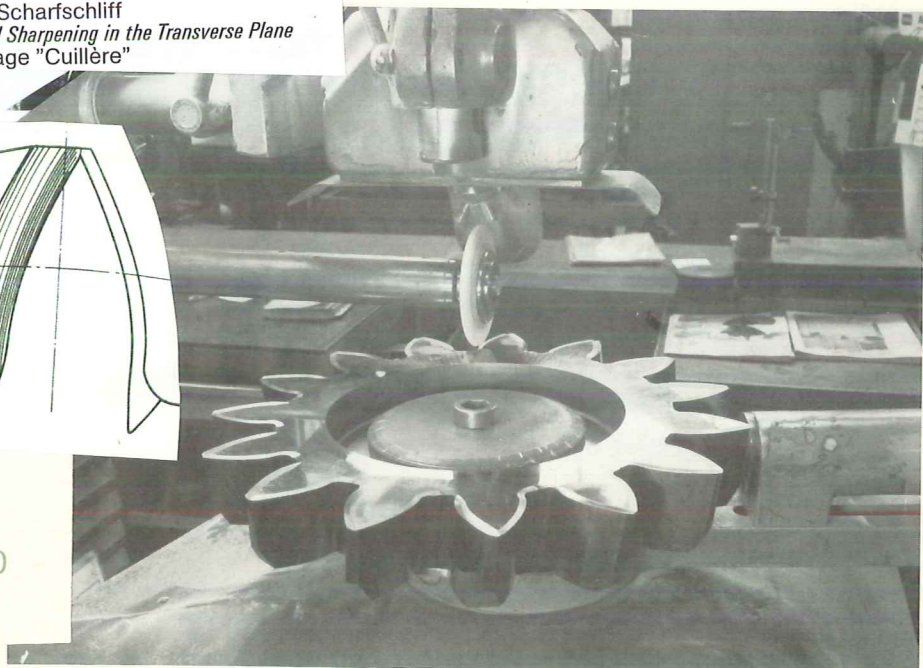
Bild 10: Schneidrad mit Stirnschliff
